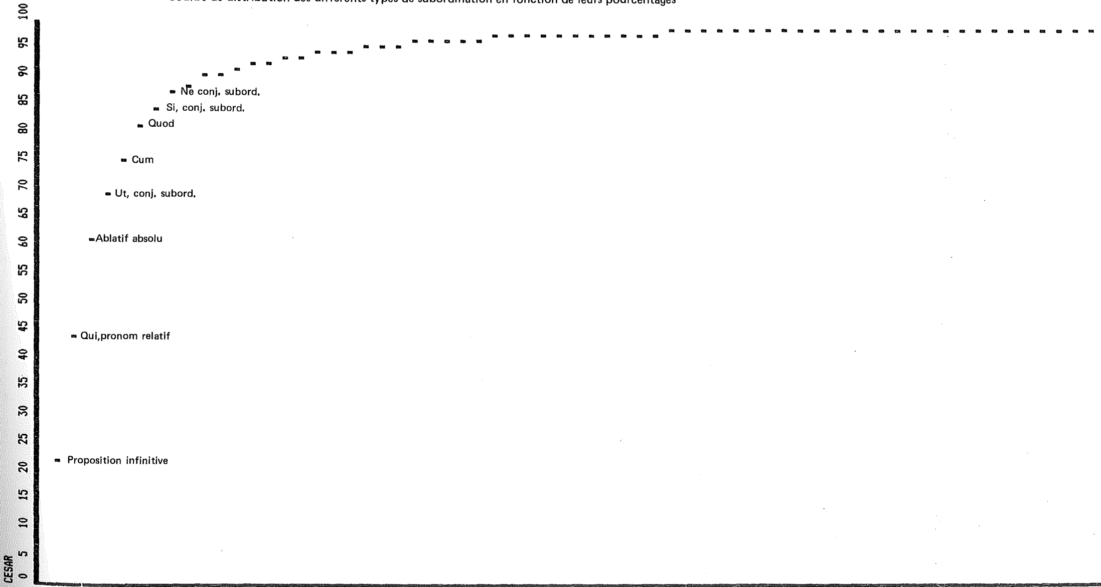
Courbe de distribution des différents types de subordination en fonction de leurs pourcentages
