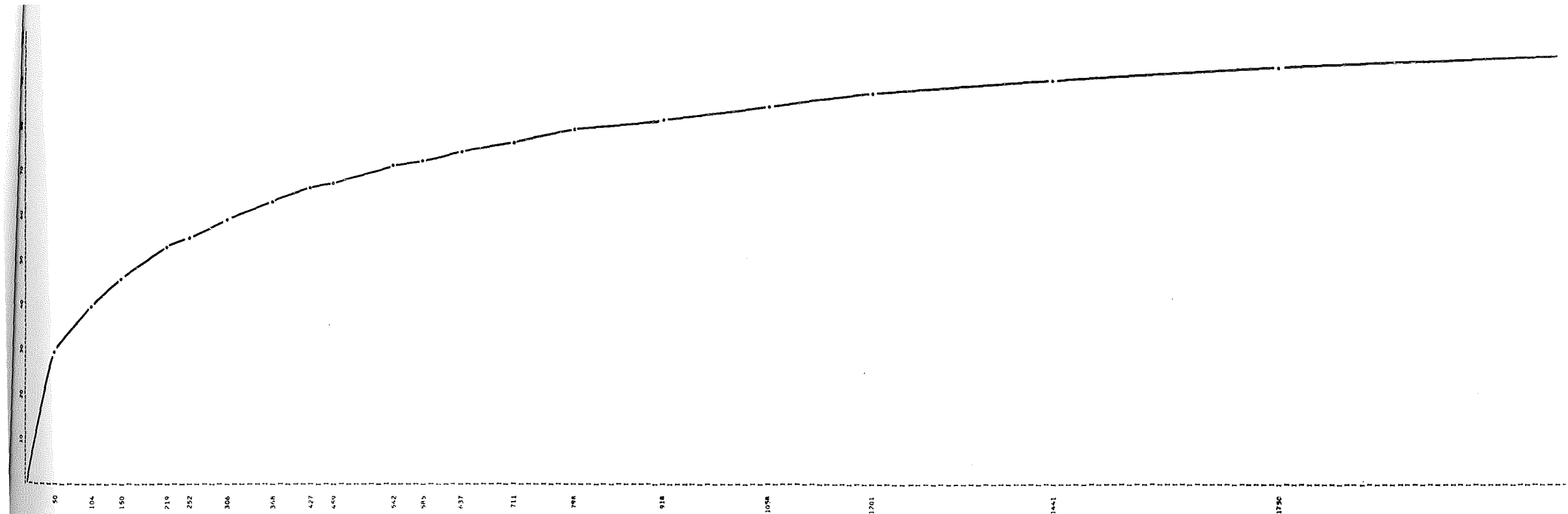
Courbe de distribution du vocabulaire de VIRGILE, Enéide
